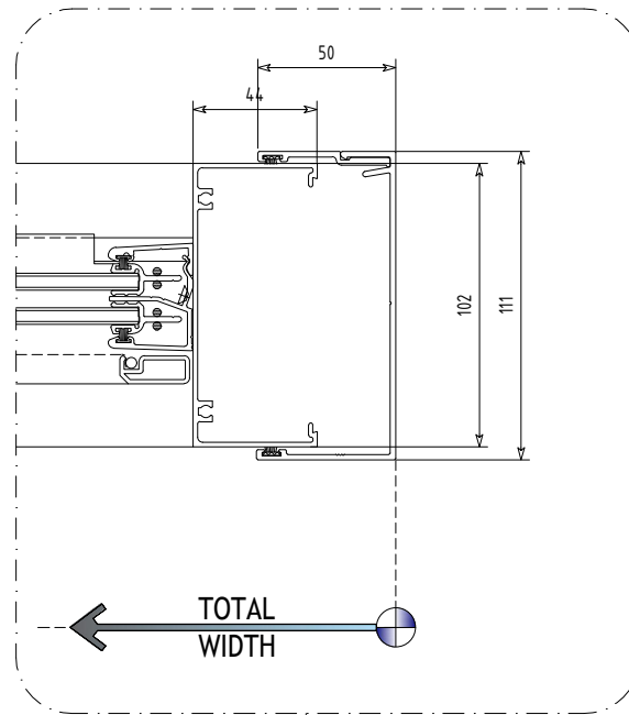
SUB-JAMB OPTION
