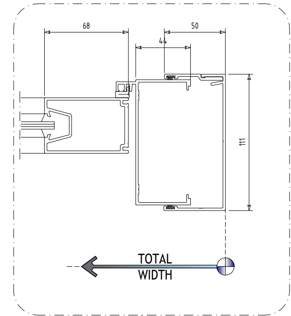
Sub-Jamb OPTION
